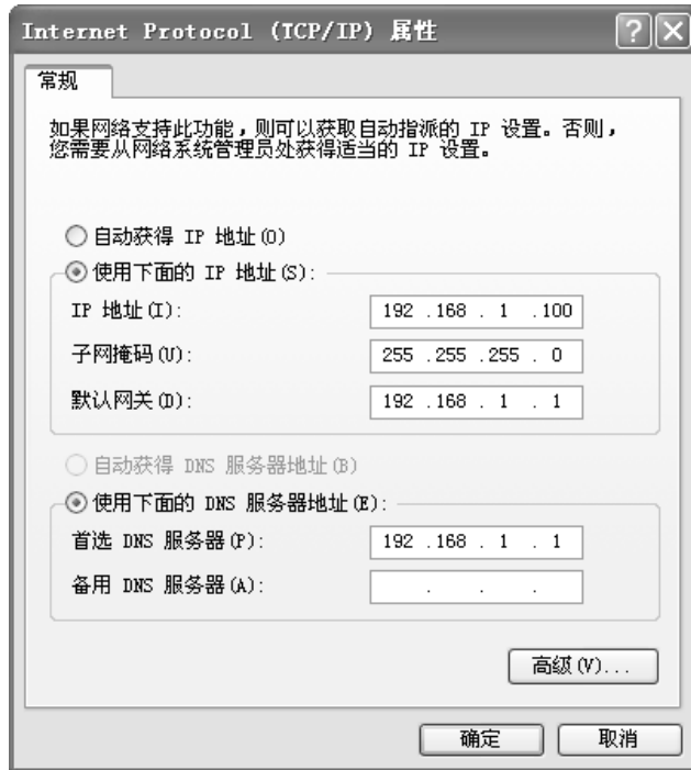
图4-1 本地连接
